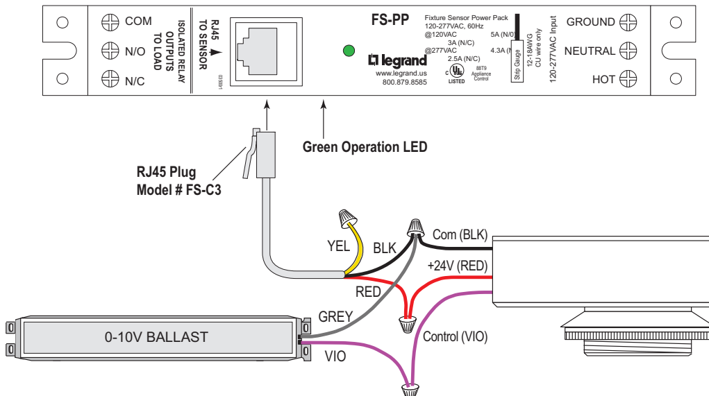
Fig 2: FS-305-D wiring
