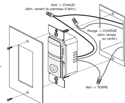
Fig. 4: Orientation du détecteur, connexions des fils et boîte murale
