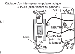
Fig. 2: Câblage d'un interrupteur unipolaire typique
